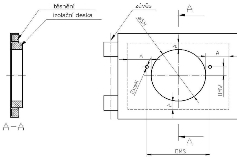
Obrázek3. Schéma provedení montážnícbtvorů pro hořáky o výkonu: 4-6 kW, 5-20 kW 6-26 kW, 8-36 kW, 10-50 kW
